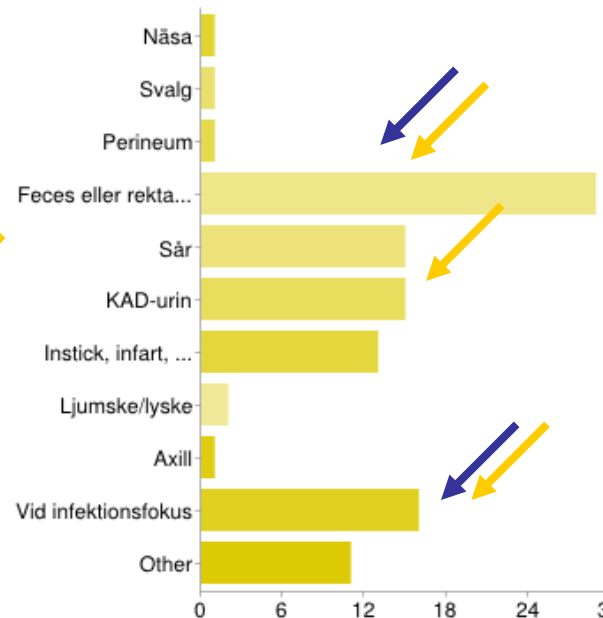
VRE
