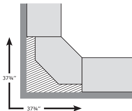
Sección de esquina con dos estructuras de 22 \frac{7}{8} " de fondo.
