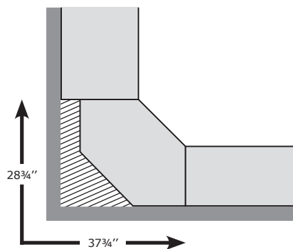
Sección de esquina con una estructura de 13 \frac{3}{4} " de fondo y otra de 22 \frac{7}{8} " de fondo.
