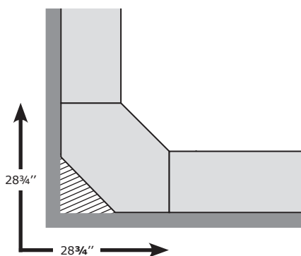
Sección de esquina con dos estructuras de 13 \frac{3}{4} " de fondo.
