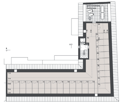
Dachgeschoss
