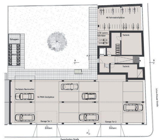
Erdgeschoss
