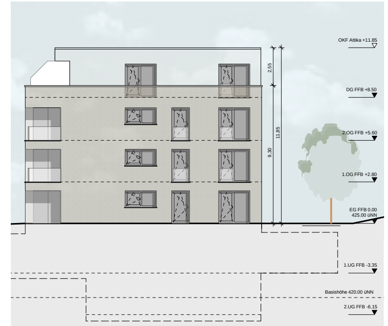
Ansicht Ost
