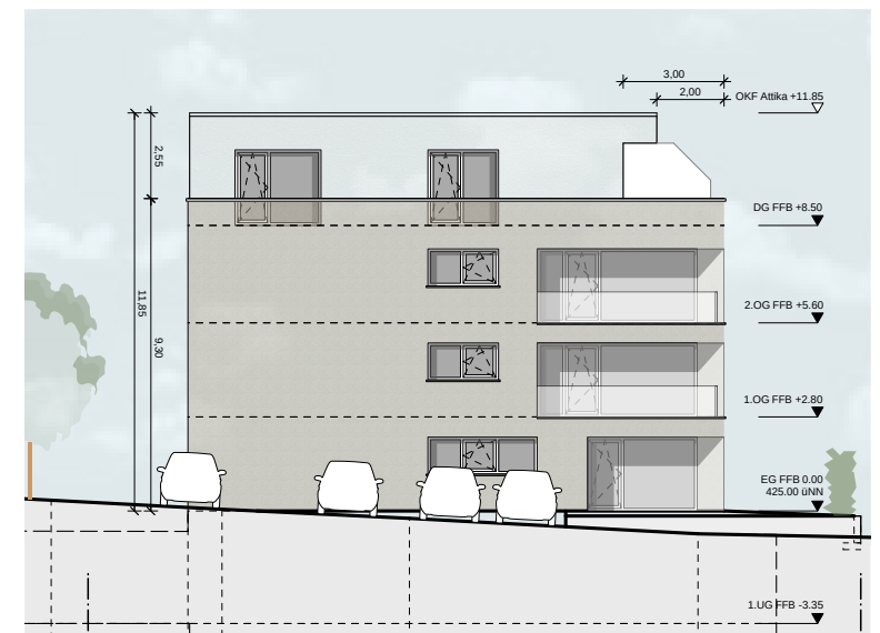
Ansicht West
