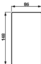
Flanschausschnitt für GHG 412 82
