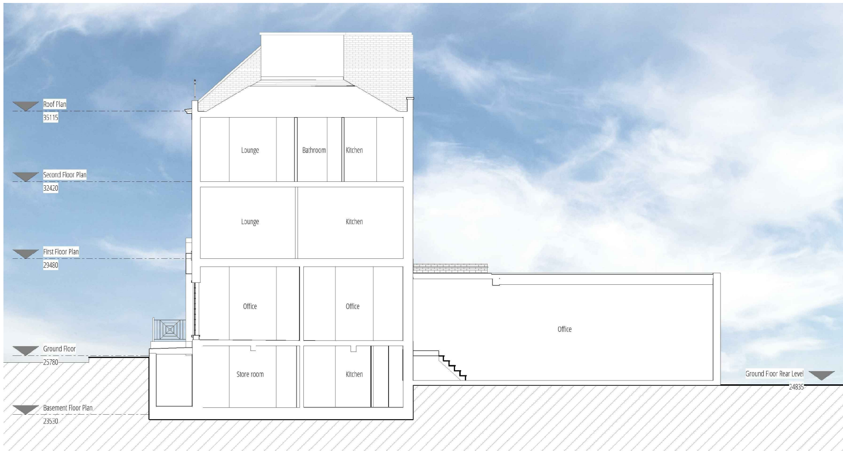
1 Existing Section EE' 1 : 100
