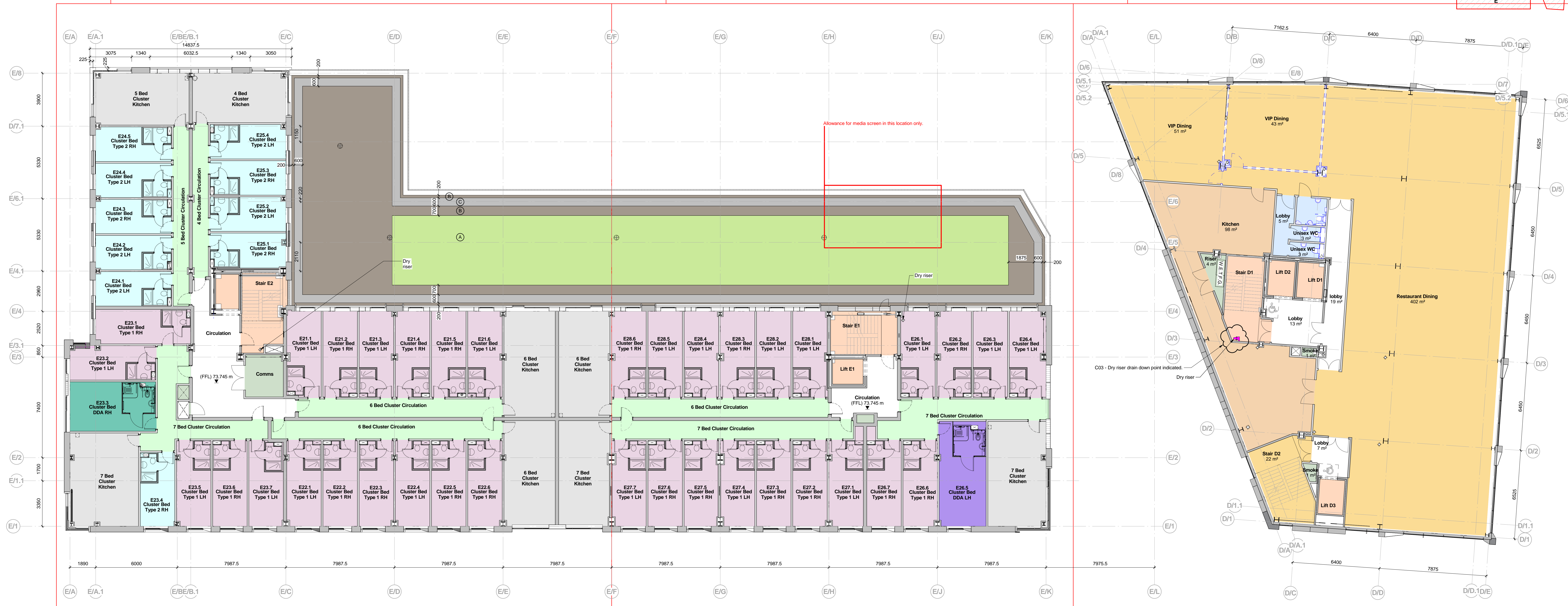
1 04 - Level 20 1 : 100
