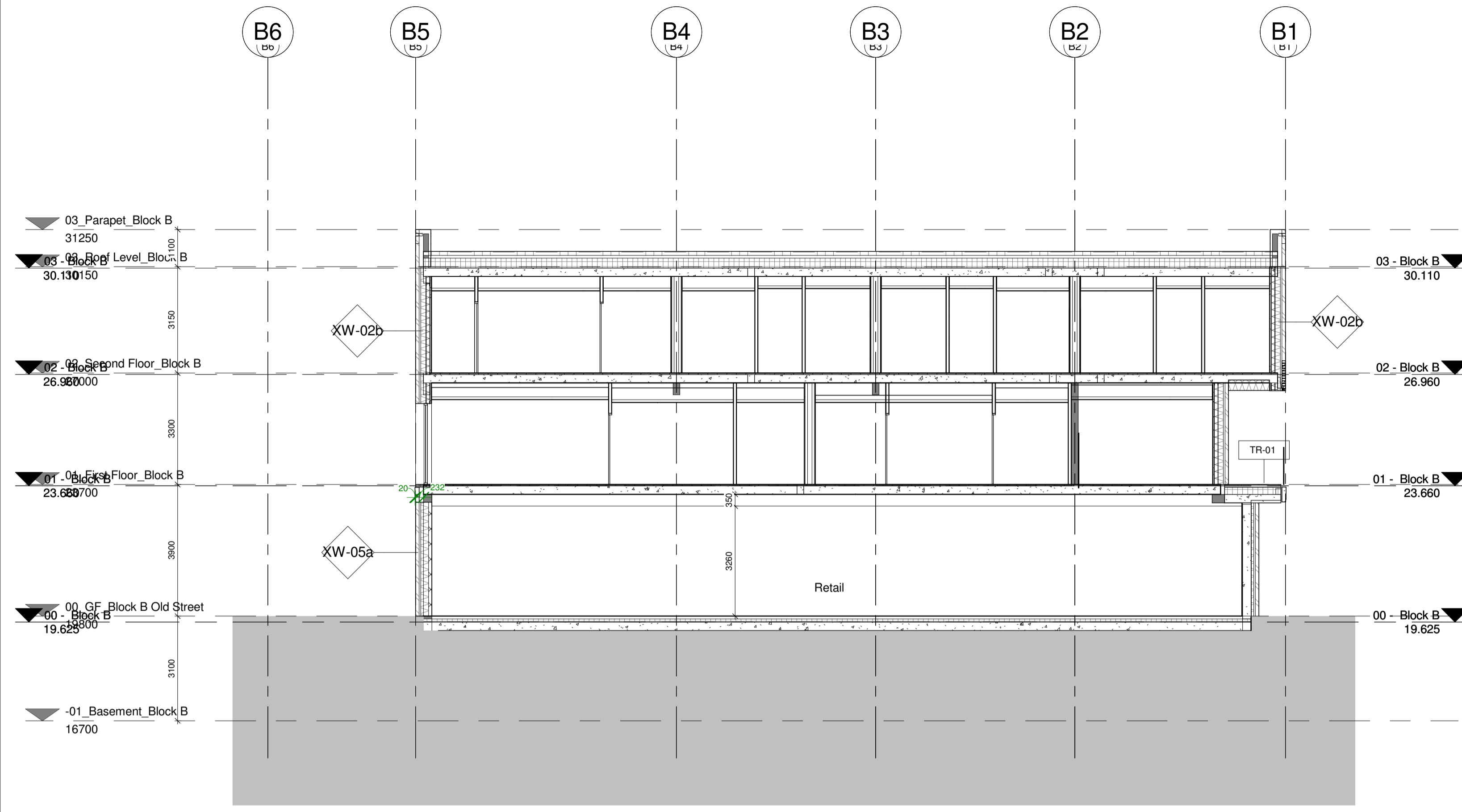
1 Block B - Section HH 1 : 100
