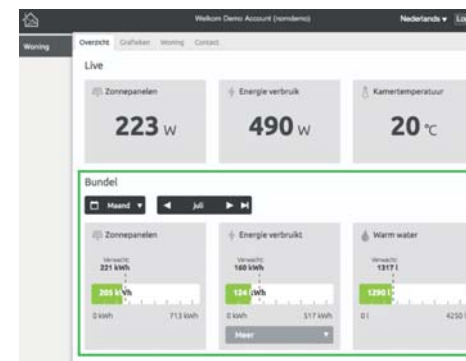
4: Bedieningsknoppen & Bundels
