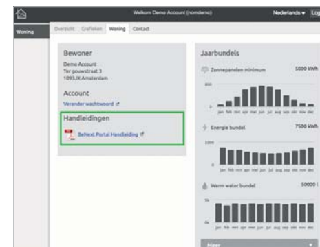
8: Handleidingen
