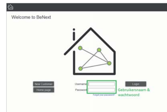
2: Loginpagina
