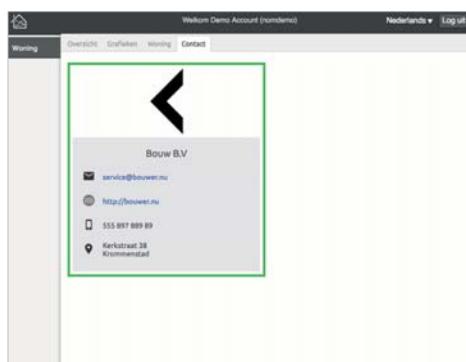
10: Contactpagina
