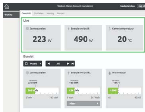
3: Live
