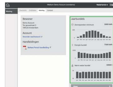
9: Jaarbundels
