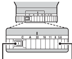
Himmenninrenkaan lukituksen vapautus Himmenninrenkas lukituksen vapautus
