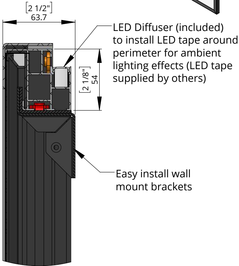
DETAIL DD SCALE 1 : 2
