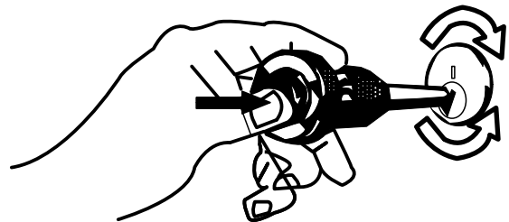
4- Kilit, kilitleme pozisyonunu çeyrek turdan daha az kala arkadaki tetikleme düğmesine basınız. Şifrelerin kilitlenmeden tütün döndüğünü göreceksiniz.
