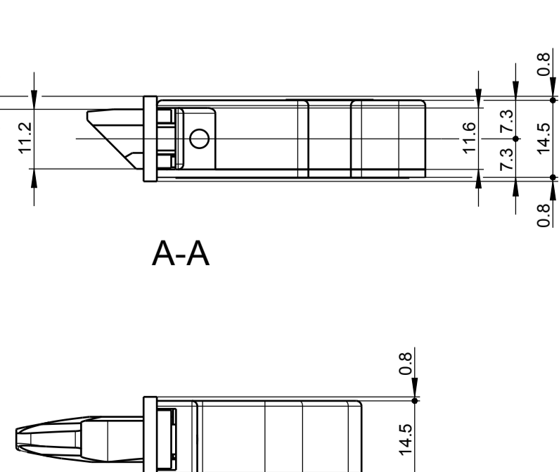
A-A
