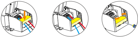
压线板
