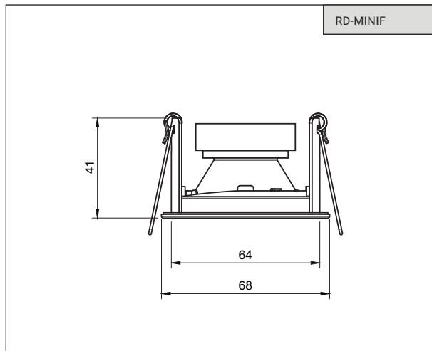
Mini Recessed Downlight
