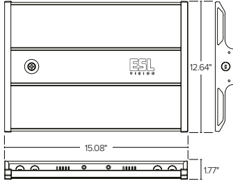
ESL-LHB-75130W-44050
