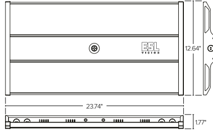
ESL-LHB-130170W-44050
