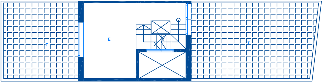
PLANTA ESTUDIO
