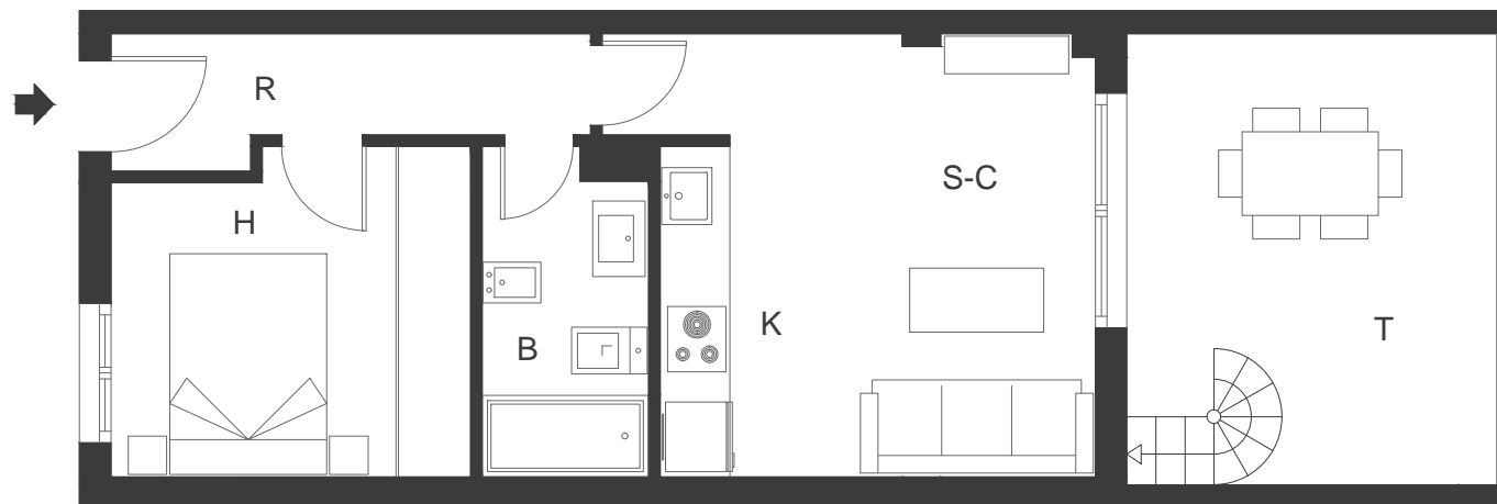
PLANTA PISO
