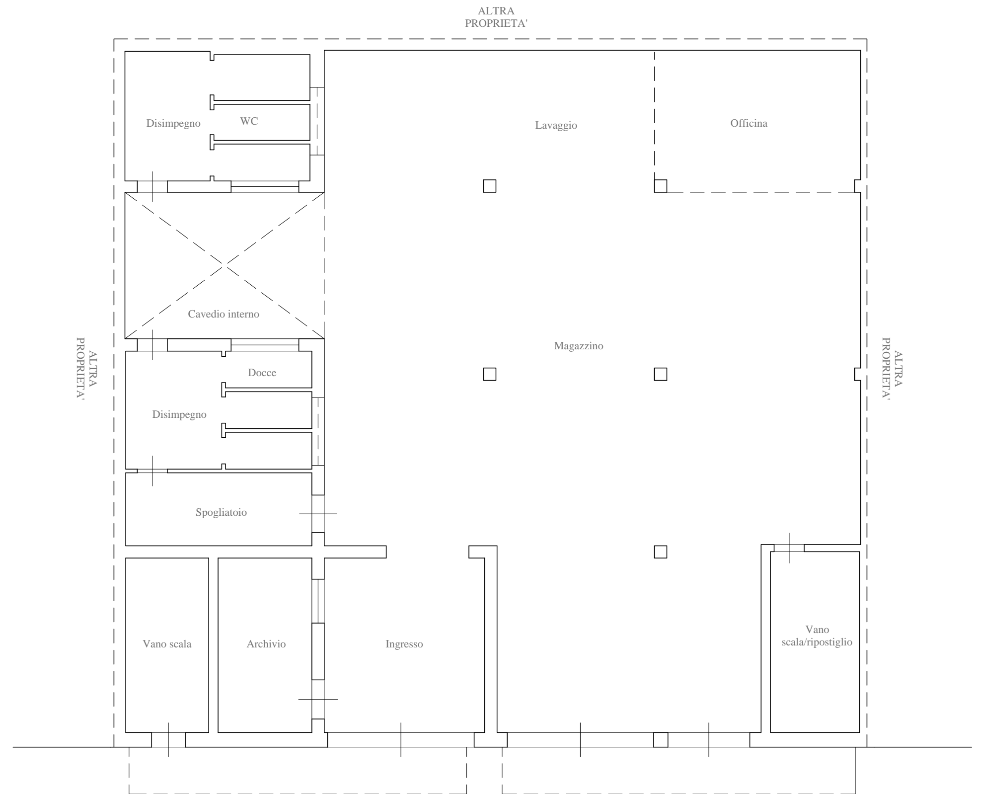
Piano Terra - Stato di Fatto
