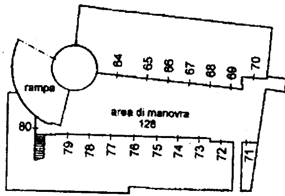
PIANO 2° SOTTOSTRADA
