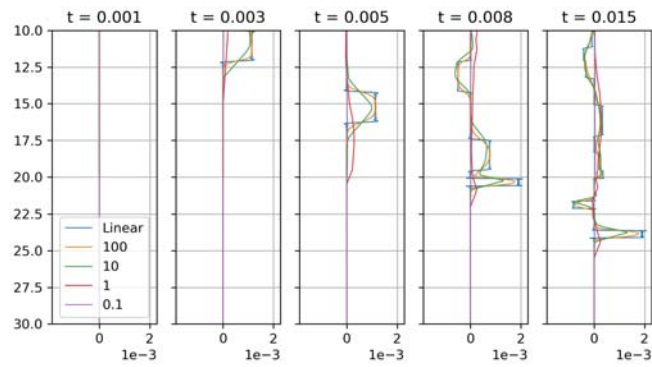
(d) Velocity of bar 2
