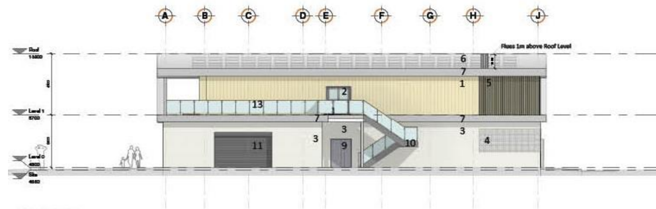
1 North Elevation Scale: 1:200
