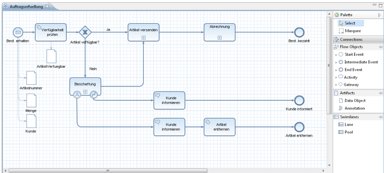
Abbildung 8.4: Beispielprozess »Auftragserfuellung« mit eingebettetem Teilprozess »Abrechnung«
