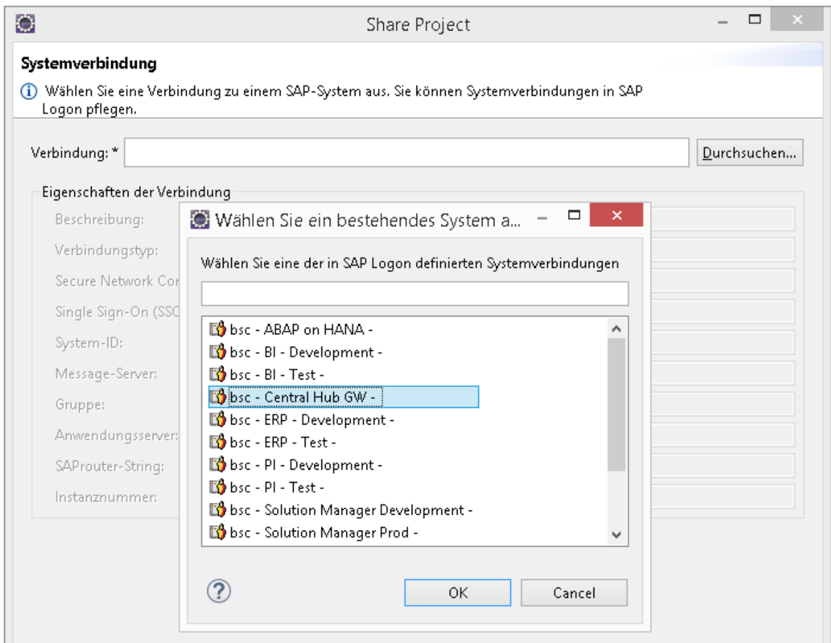
Abbildung 5.35: Backend-System auswählen
