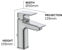
Tesi Basin Mixer
