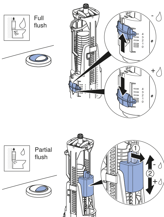
Flush valve (Typ 240)
