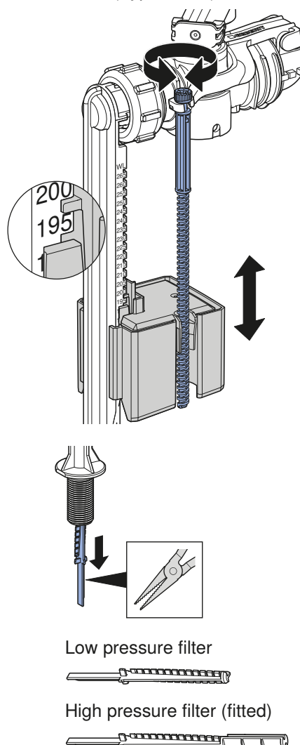
Fill valve (Typ 380AG)
