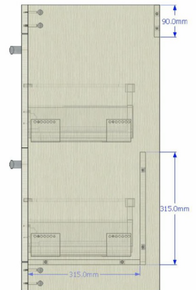
Right Elevation
