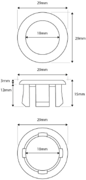
Dimensions
