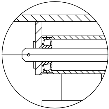
Gelagerd Zwenkpunt (Rotation point with ball bearing)
