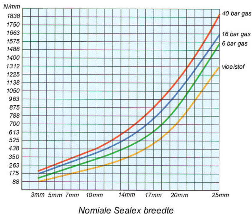
Aanbevolen montage vlakke per lengte Sealex
