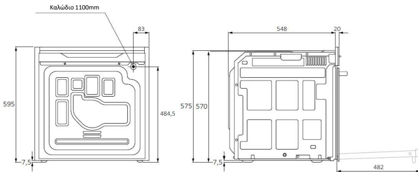
Οπίσθια όψη
