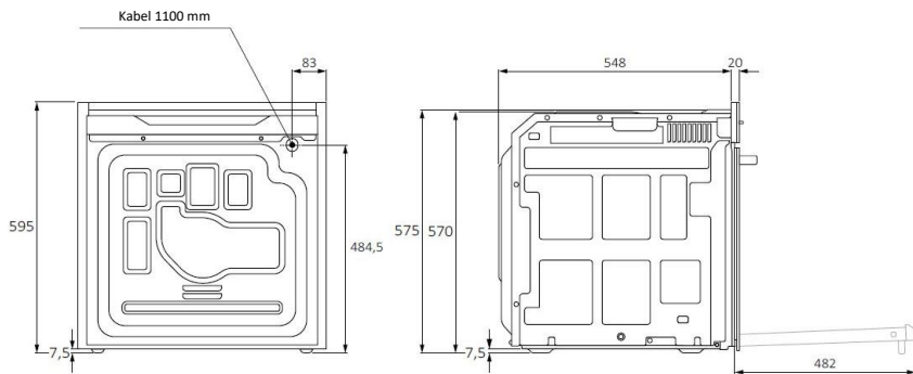
Achteraanzicht
