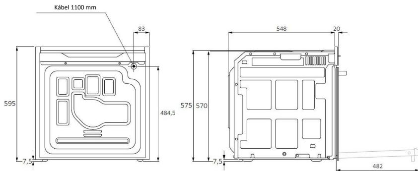
Pohľad zozadu
