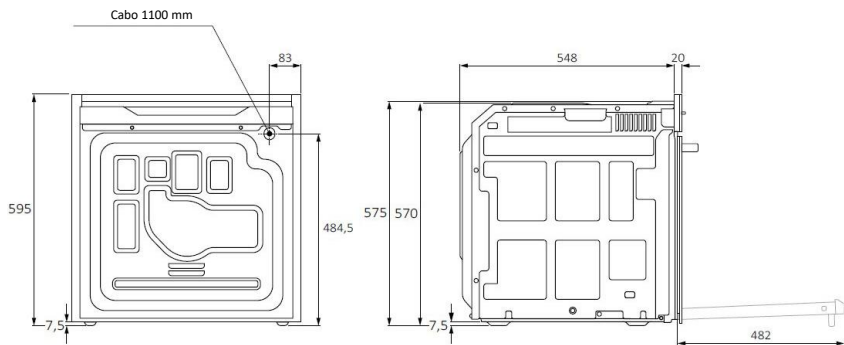
Vista posterior
