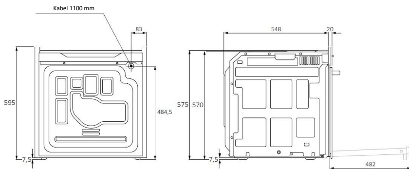
Vista posteriore
