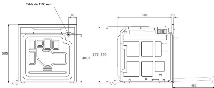
Vista posterior
