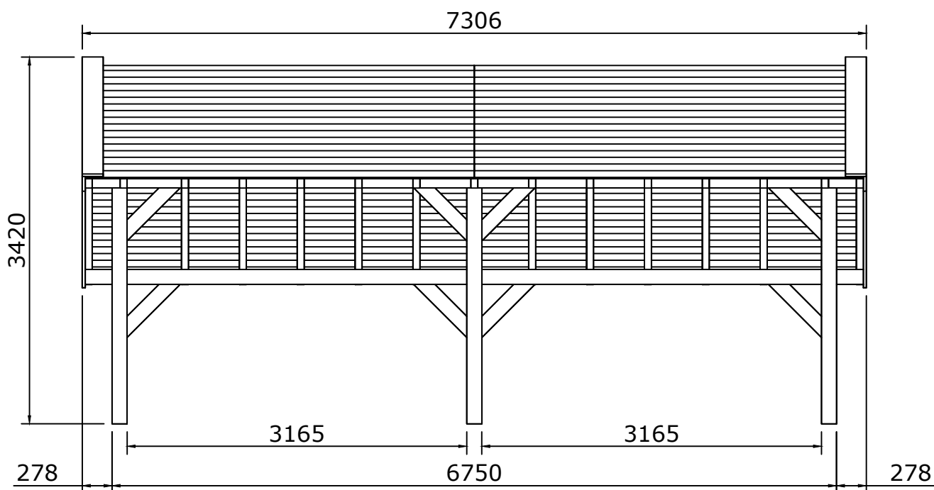
Vooraanzicht - Front view - Vorderansicht
