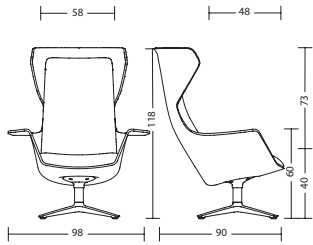
woo75 mit Armlehnen: woo75 - 20 kg
