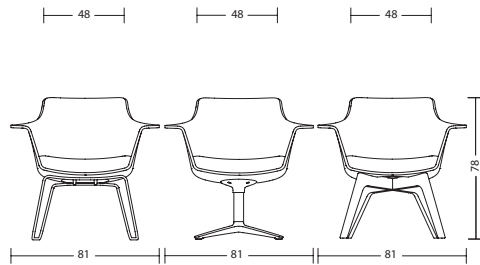
woo58 + 3246 / 3231 / 3206 mit Armlehnen: woo58 - 8 kg
