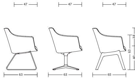
woo58 + 3246 / 3231 / 3206 mit Armlehnen: woo58 - 8 kg
