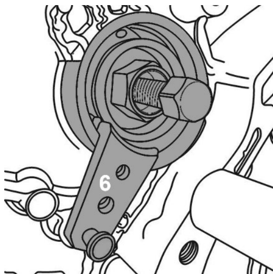
3. Extracteur de pompe haute pression diesel (6), à utiliser comme OEM 654 589 00 14 00
