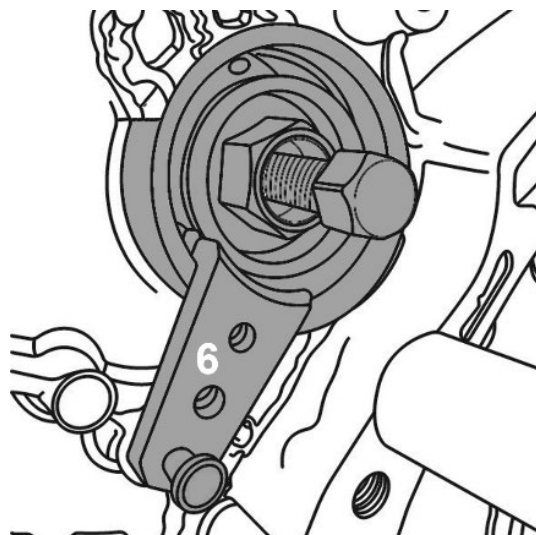
3. Extractor de bomba de alta presión diésel (6), para usar como OEM 654 589 00 14 00
