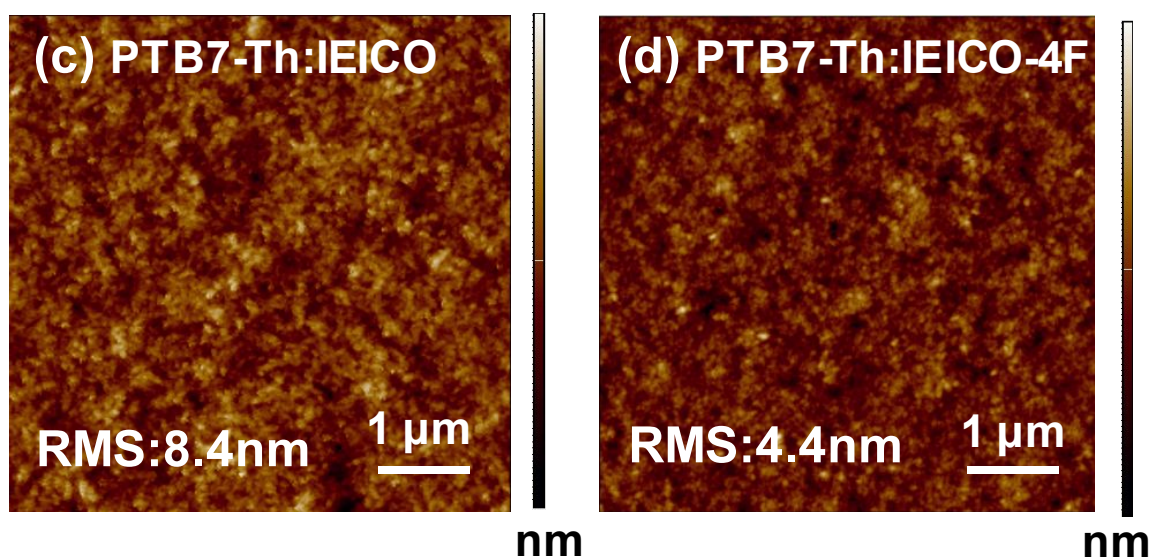
Figure S3 AFM height images (5 μm×5 μm) of (a) PBDB-T:ITIC, (b) PBDB-T:IT-4F, (c) PTB7-Th:IEICO and (d) PTB7-Th:IEICO-4F films.
