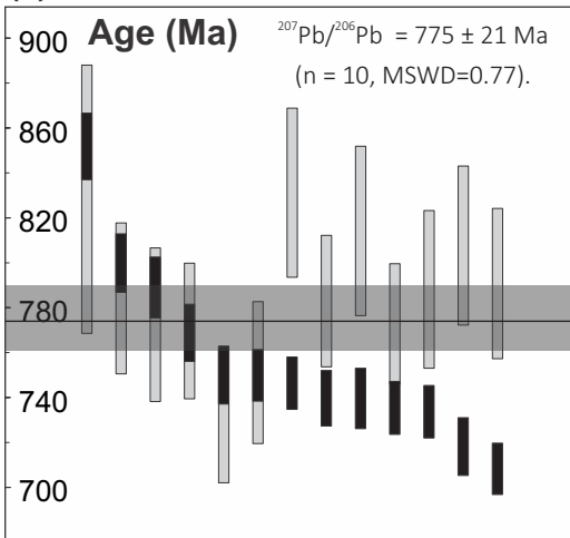
(d) AJ14-23: Microgranodiorite
