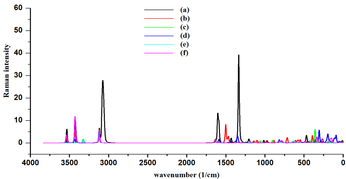
Fig.S4.2 Raman spectrum of (a) G-CA (b) F-CA (c) AlN-CA (d) AlP-CA (e) BN-CA (f) BP-CA
