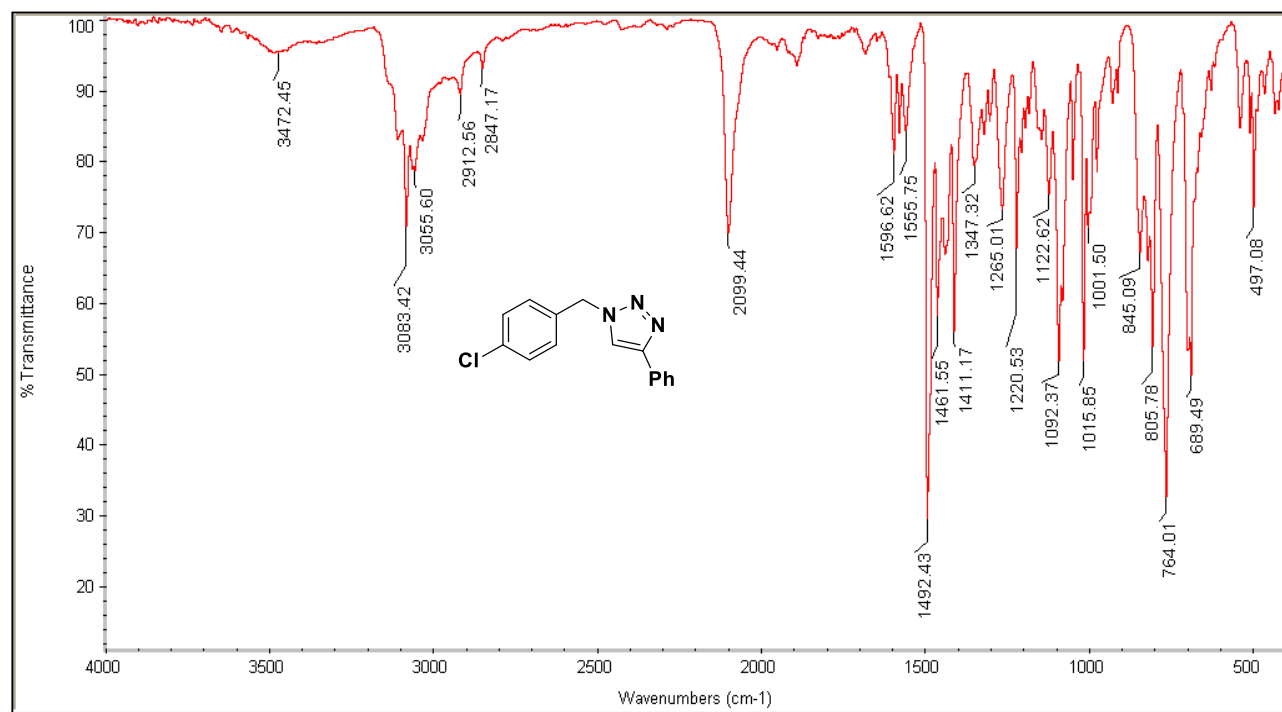
Fig. S6 FT-IR of 1-(4-chlorobenzyl)-4-phenyl-1 H -1,2,3-triazole ( 5d , 5e , Table 3, Entries 4,5)
