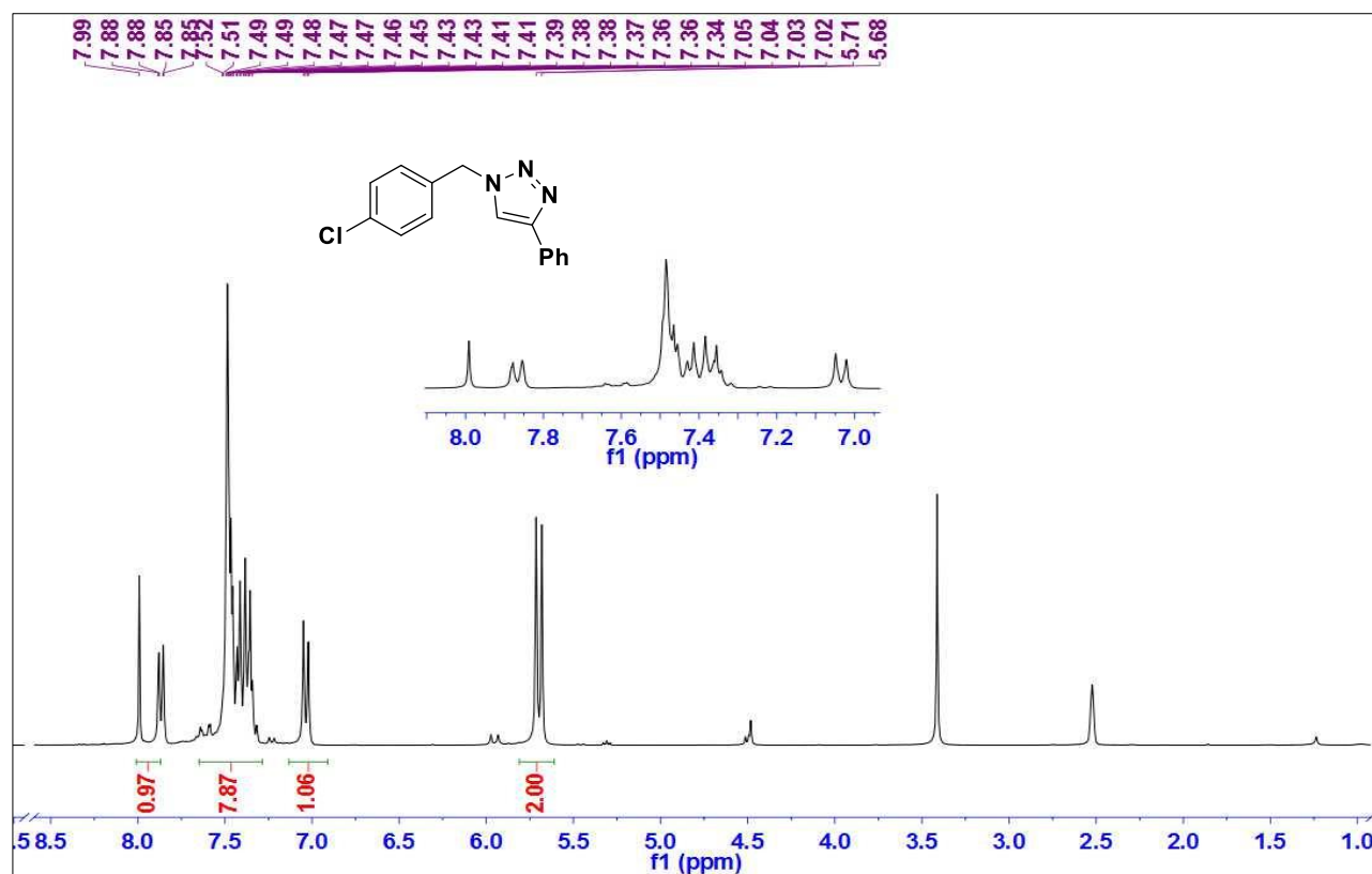
Fig. S7 1 H-NMR of 1-(4-chlorobenzyl)-4-phenyl-1H-1,2,3-triazole ( 5d , 5e , Table 3, Entries 4,5)
