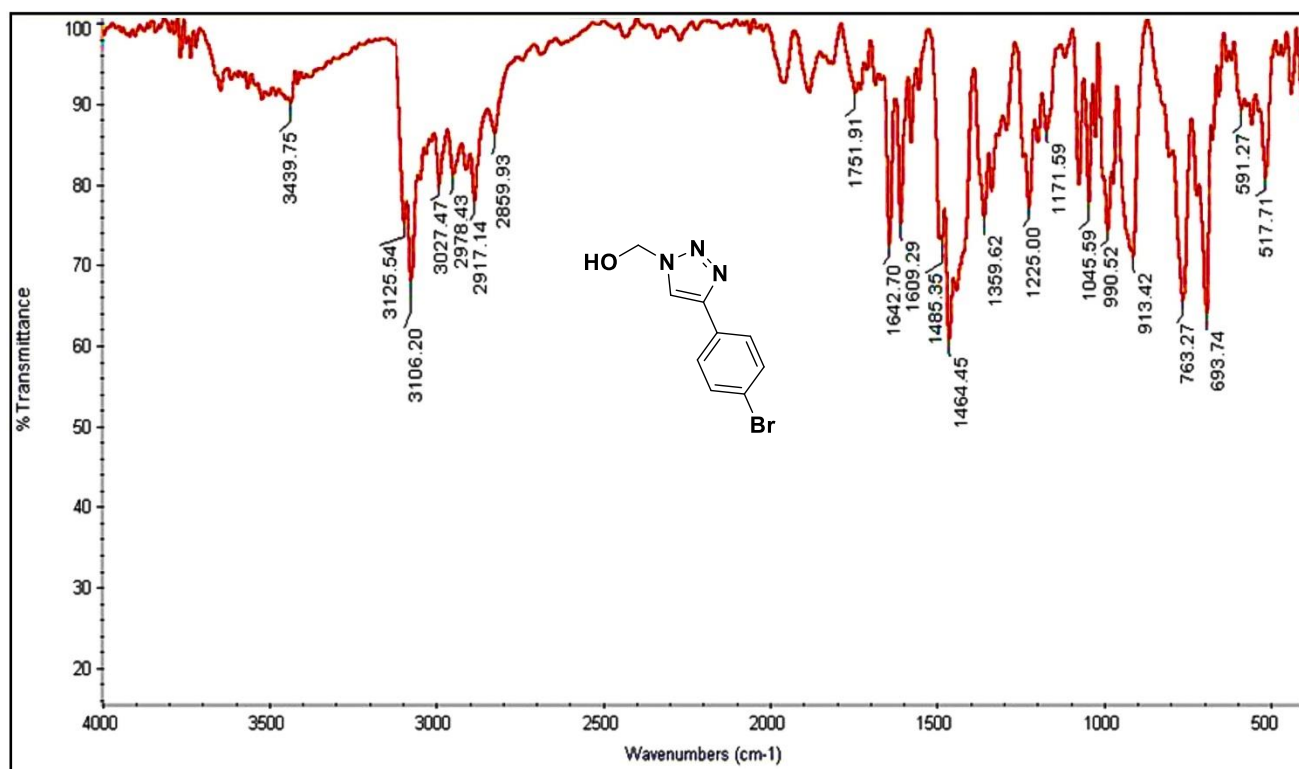
Fig. S17 FT-IR of (4-(4-bromophenyl)-1 H -1,2,3-triazol-1-yl)methanol ( 6h , Table 3, Entry 16)
