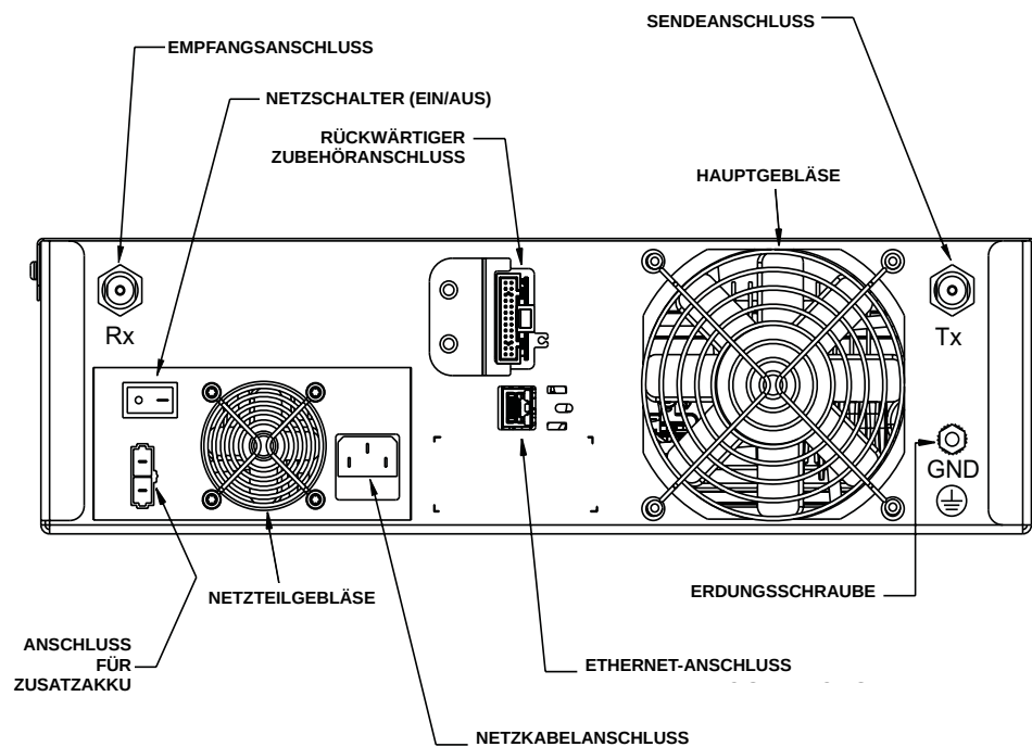
Abbildung 4-1 Anordnung der Anschlüsse auf der Rückseite des Repeaters
