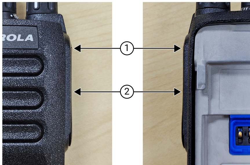
Figure 2 : Le couvercle antipoussière est fixé
