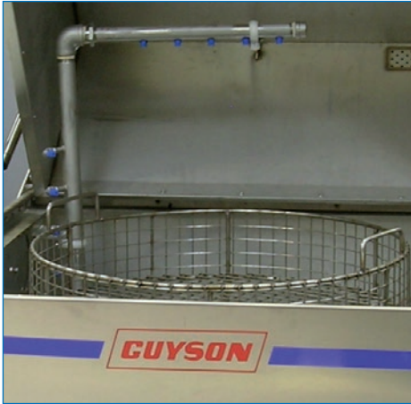
Barres de pulvérisation en haut, sur les côtés et en bas
