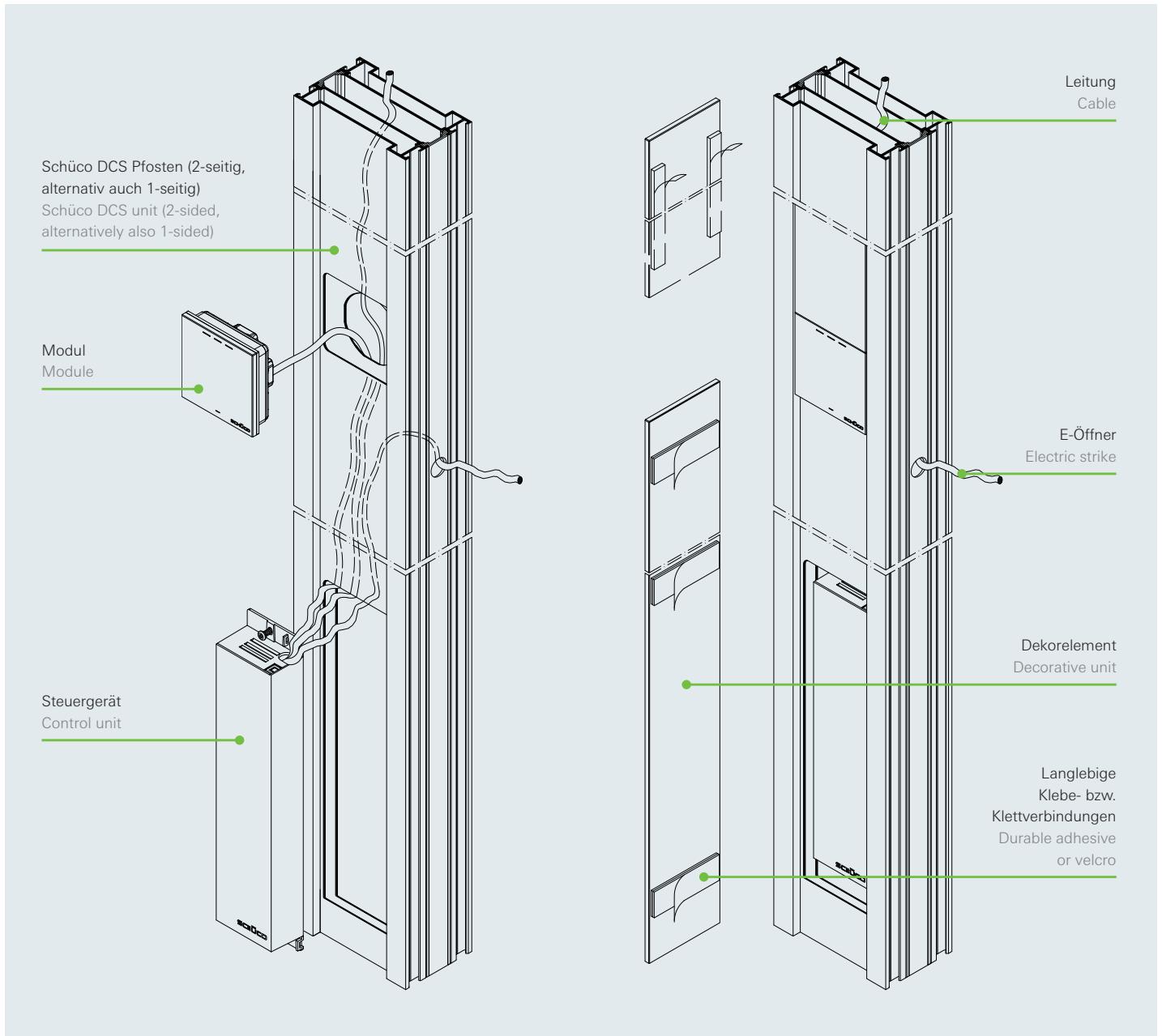
Schüco DCS Pfosten (2-seitig) für die Zutrittskontrolle Schüco DCS unit (2-sided) for assignment control
