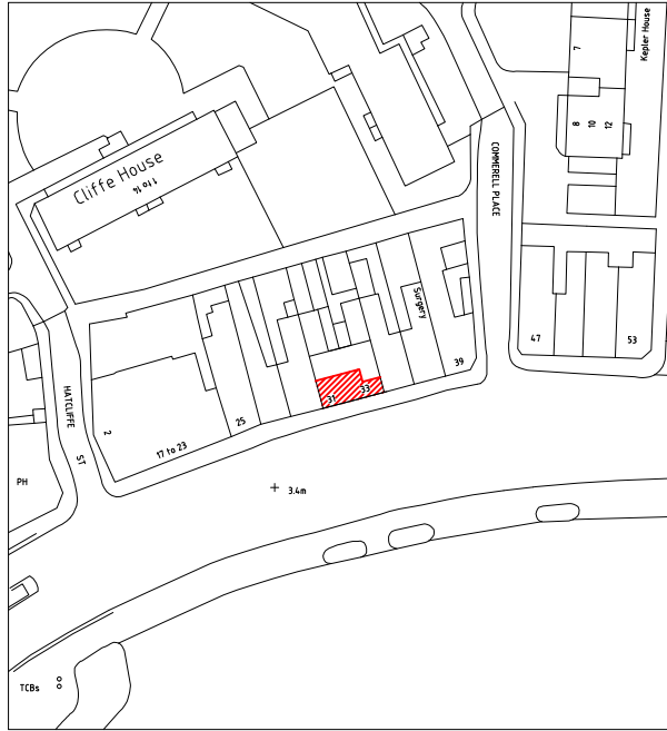
Site Plan 1:1250
