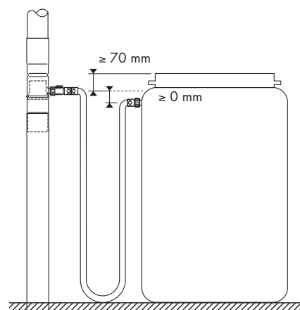
Korrekt montage og opstilling
