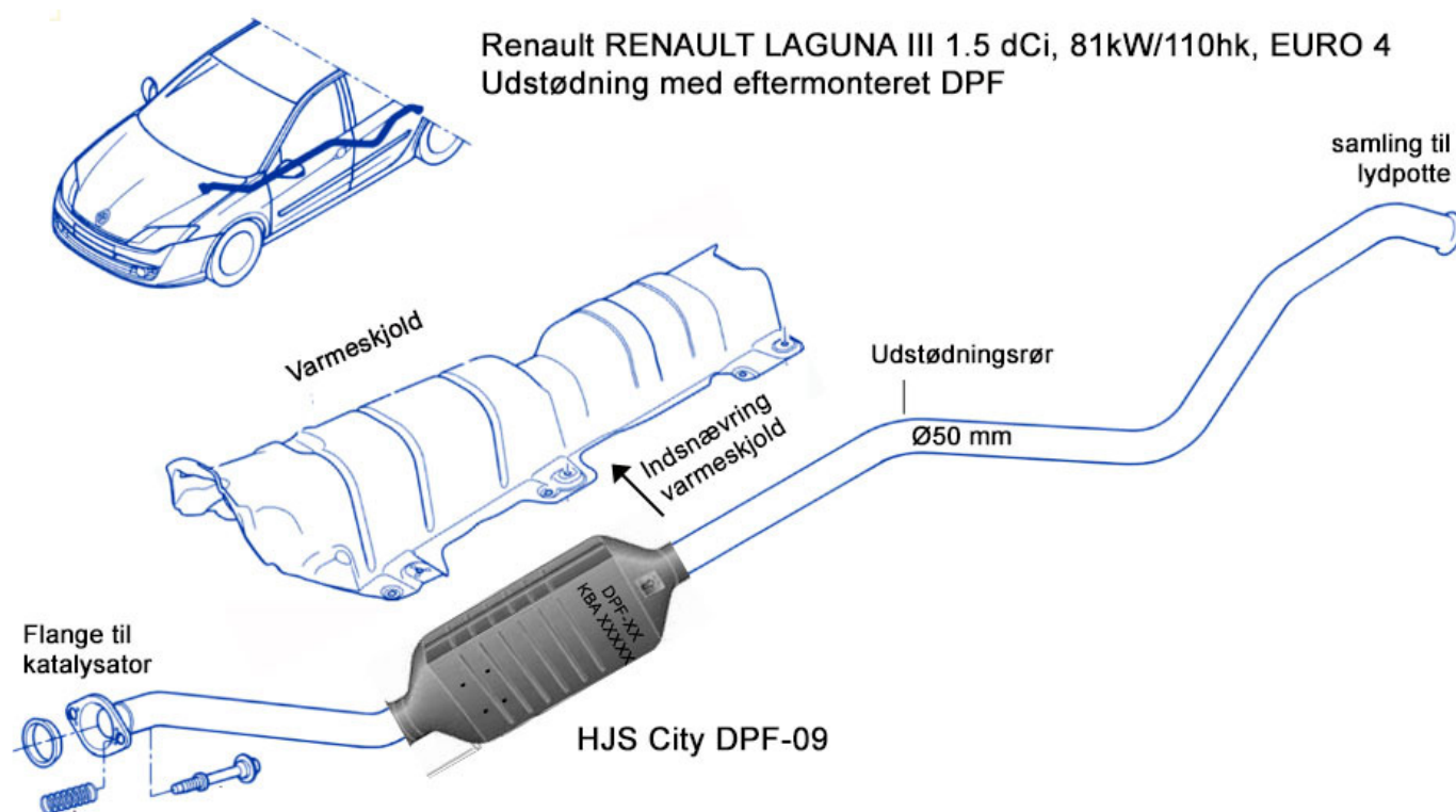
Modificeret udstødning med DPF monteret imellem ophæng og flangesamling.
