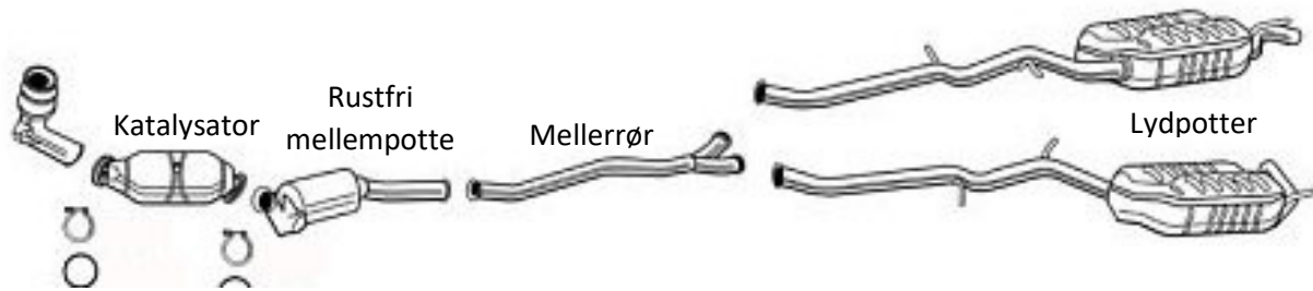
Original udstødning – forrør, 2 katalysatorer, mellemrør og lydpotter.
