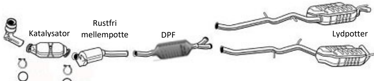
Modificeret udstødning med DPF monteret på mellemrør.
