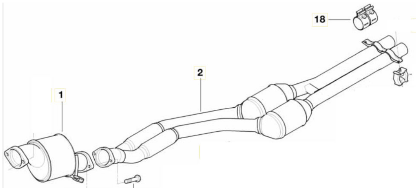
Originalt for-katalysator(1) og 2 parallelle katalysatorer på forrør (2). Partikelfilteret erstatter de 2 katalysatorer på forrør.
