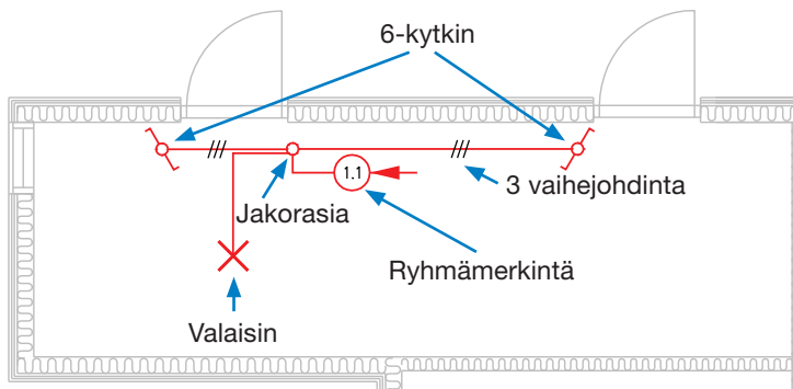
Kuva 3.40 6-kytkimien ohjaama valaisin asennuspiirustuksessa.
