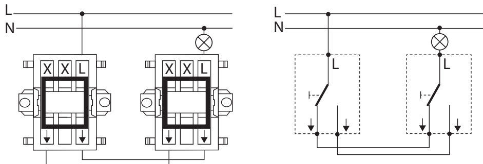
Kuva 3.39 6-kytkimen kytkentäkaavio.
