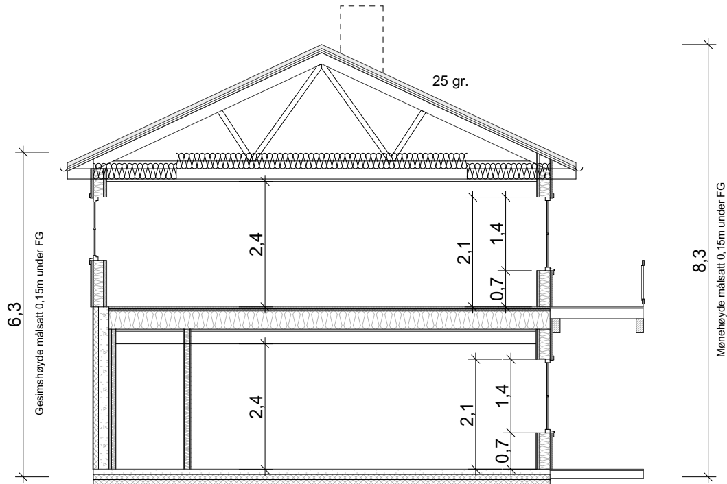
SNITT A - A
