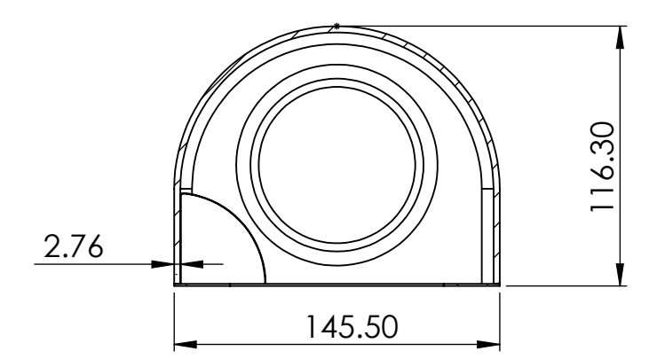
COUPE A-A
